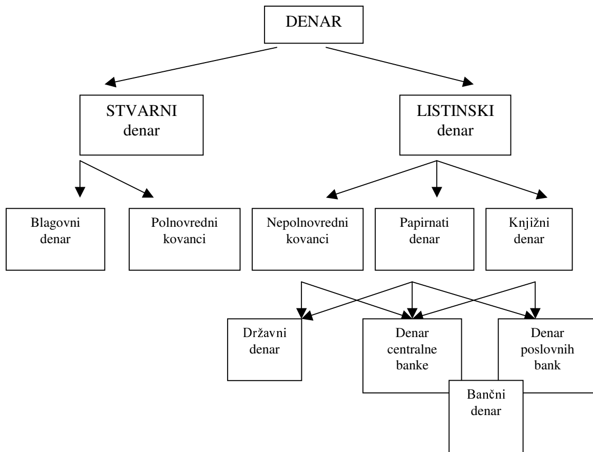
Slika 3.1 Klasifikacija denarja
